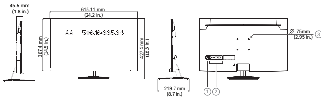
Abb. 1: Abmessungen Hochleistungs-LED-Monitor (27 Zoll)
