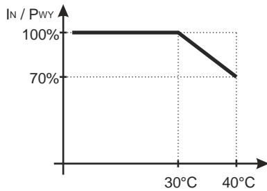
Schaubild 1: Zusammenhang zwischen Umgebungstemperatur und Ausgangsstrom
