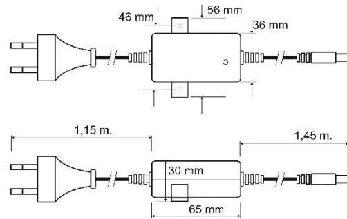
Abb. 1: Abmessungen
