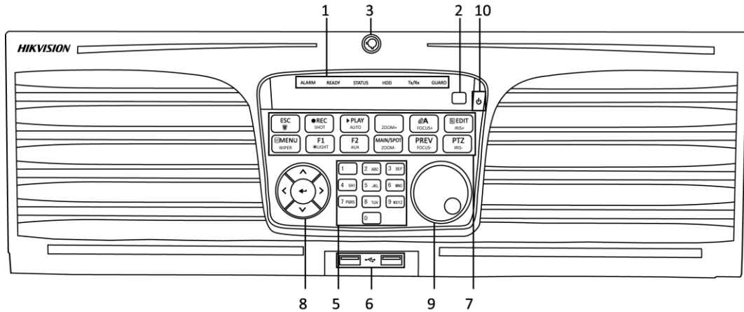
Abbildung 1-2 DS-9600NI-I16 Serie
