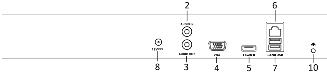
Abbildung 1–14 DS-7600NI-K1 Serie
