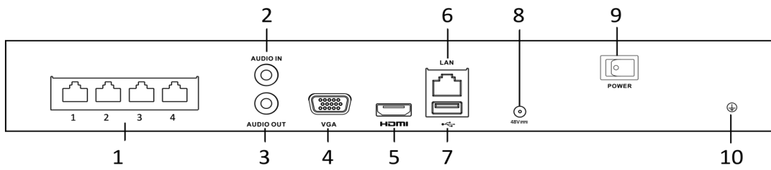
Abbildung 1–15 DS-7604NI-K1/4P Serie
