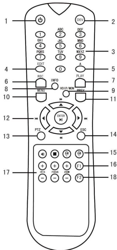
Abbildung 1–7 Fernbedienung
