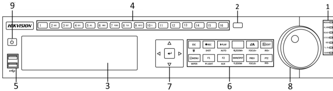
Abbildung 1–3 DS-8600NI-I8 Serie
