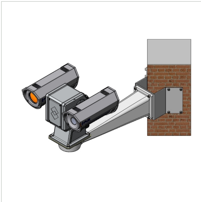
PT-CRNR-00 Eckbefestigung, für FLIR PT-Serie
